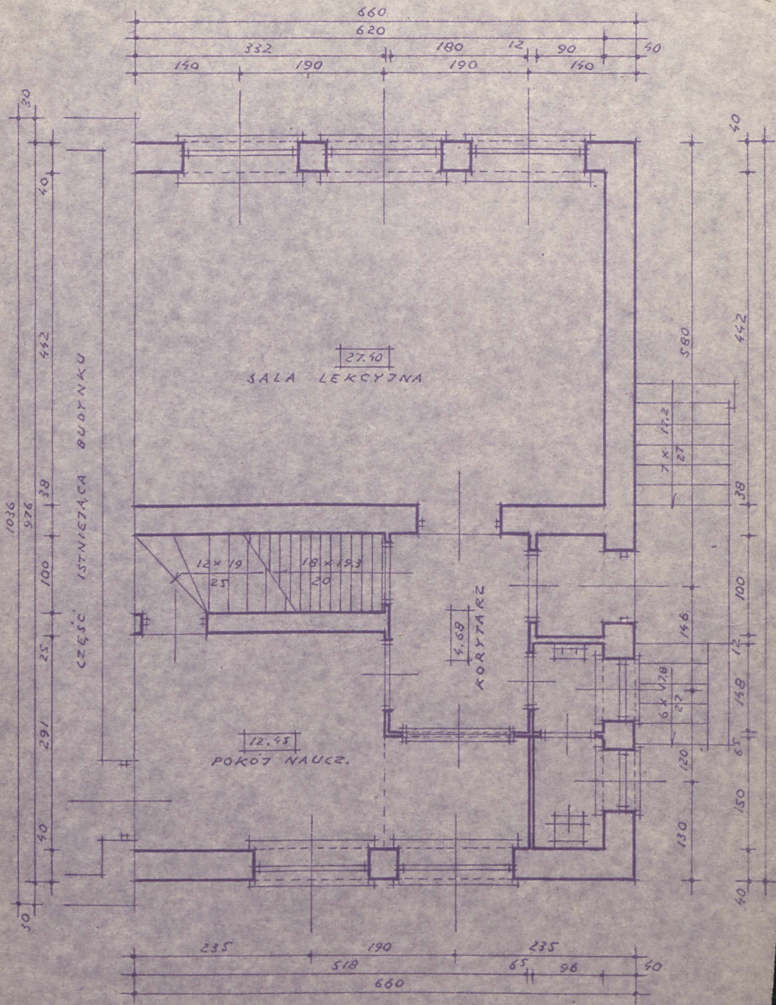
RZUT POZIOMY PRZYZIEMIA 1-50
