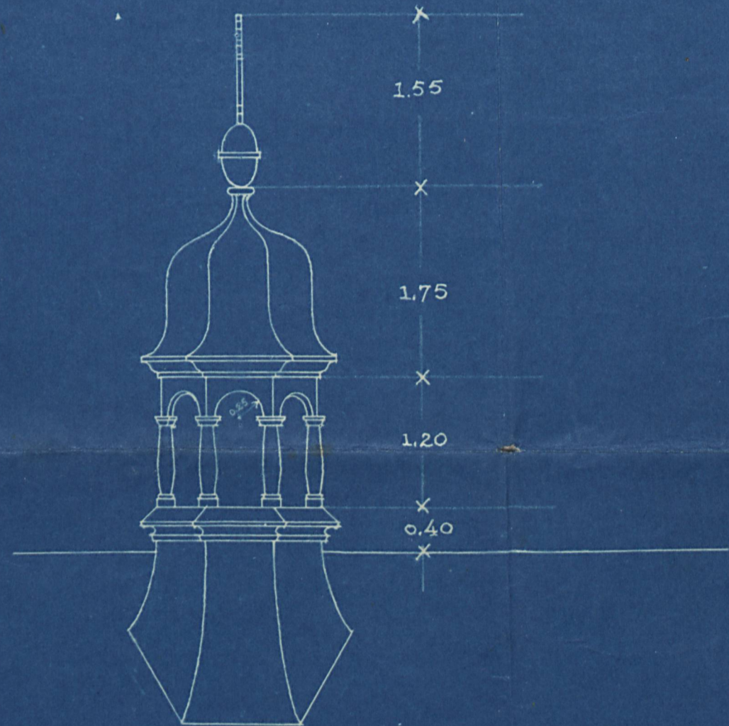
SYGNATYBKA, 1:50
