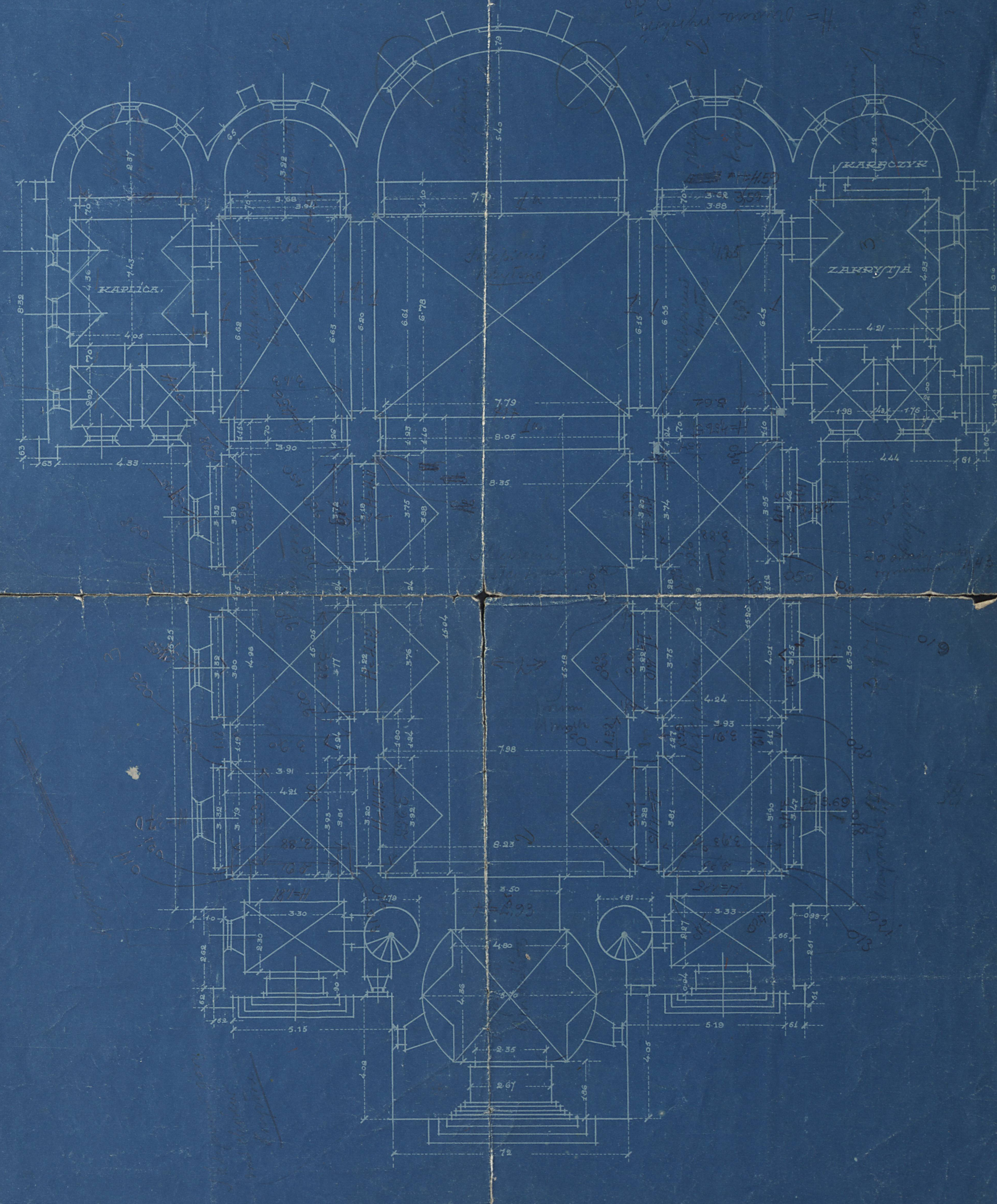
POZIOMKA 1:100
