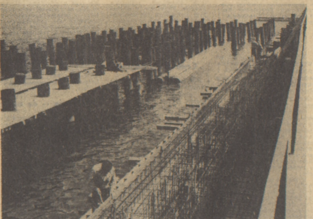
Baza rudy w Porcie Północnym. Trwają roboty zbrojarskie przy pierze. Wykonuje je brygada Maksymiliana Jabłońskiego. (P)
