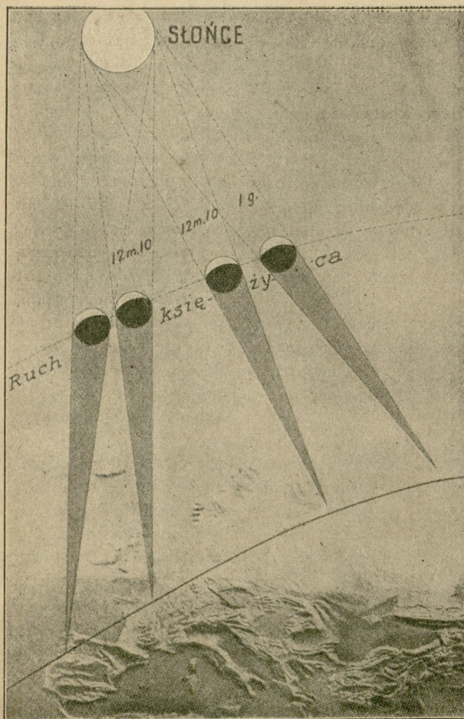
Ruch księżyca w czasie zaćmienia słońca.
